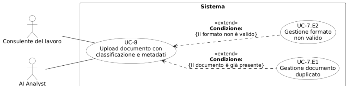
Figura 42: Diagramma del caso d’uso UC-8: Caricamento documento con classificazione e metadati manuali
