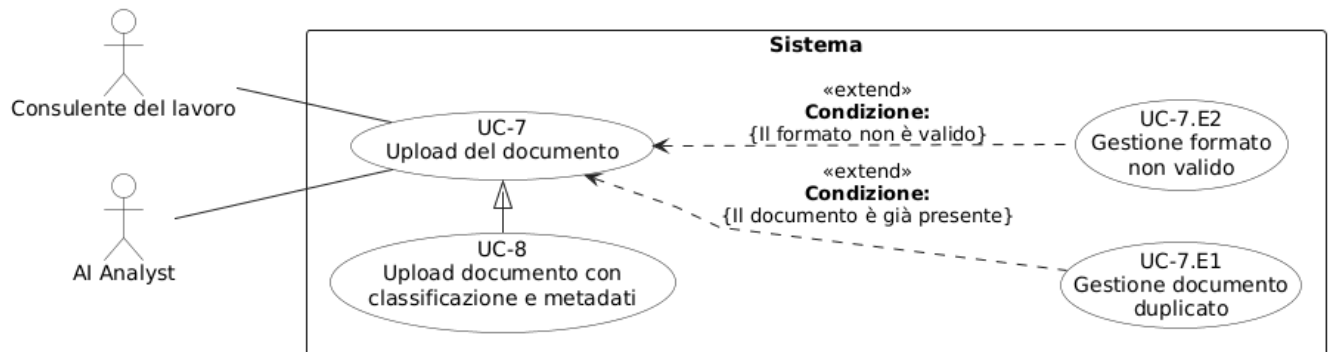
Figura 39: Diagramma del caso d'uso UC-7: Caricamento documento per analisi AI automatica
